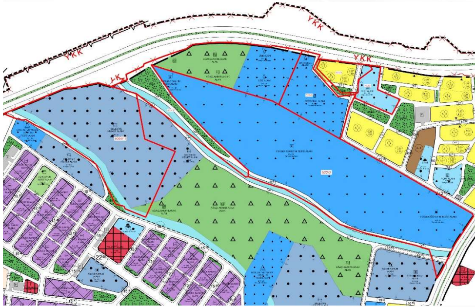
İmar Plan Değişiklik Öncesi Durum 1/1000 Uygulama İmar Planı
